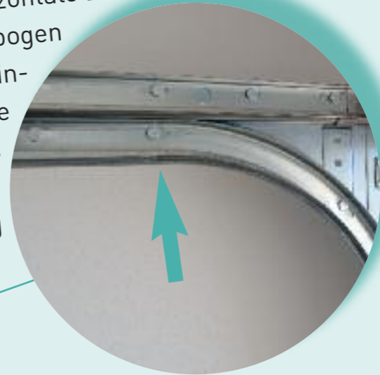
Seitlich komplett geschlossenes Zargensystem mit optimalem Eingreifschutz, der auch den oberen Schienenbogen mit absichert
