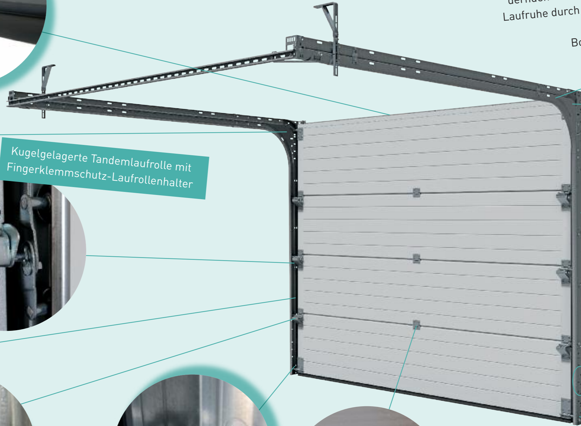
Doppellippendichtung bei der Zarge
